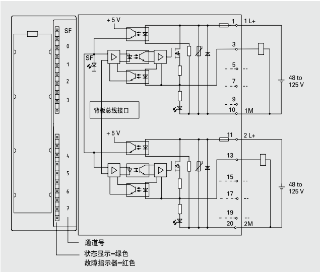
数字输出模块 SM 322; DO 8 x 48-125 VDC/1.5A 订货号: 6ES7322-1CF00-0AA0
