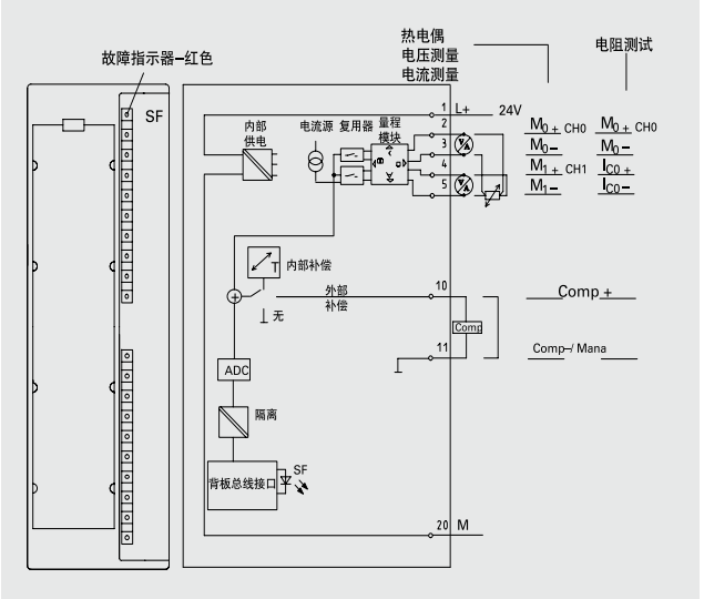
模拟量输入模块 SM 331 AI 2 x 12位 订货号: 6ES7331-7KB02-0AB0
