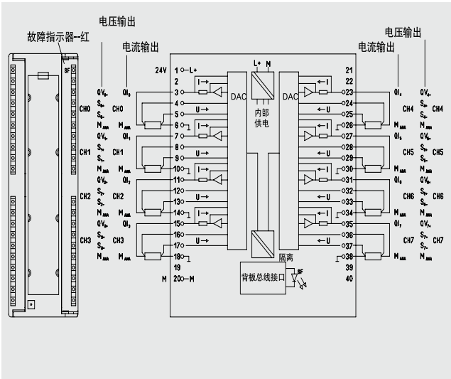
模拟量输出模块 SM 332 AO 8 × 12位 订货号: 6ES7332-5HF00-0AB0
