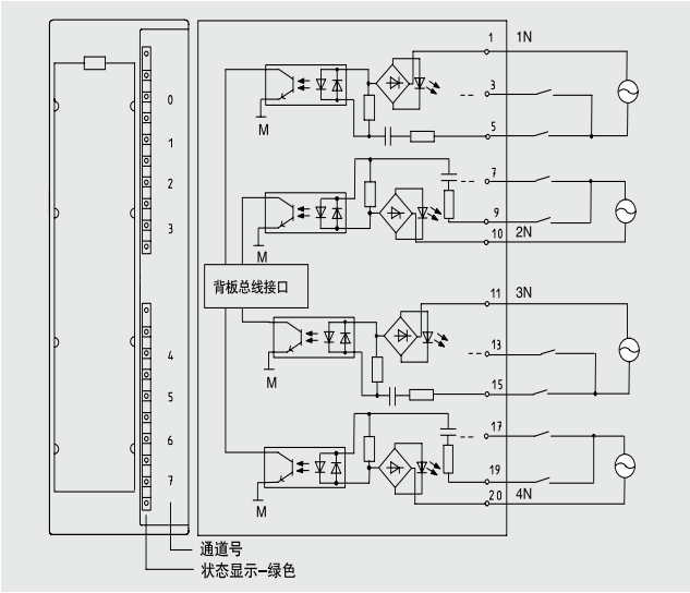
数字输入模块 SM 321 ;DI 16 X 120/230 VAC 订货号:6ES7321-1FF01-0AA0
