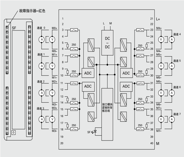
模拟量输入模块 SM 331 AI 8 x 16位 订货号: 6ES7331-7NF00-0AB0
