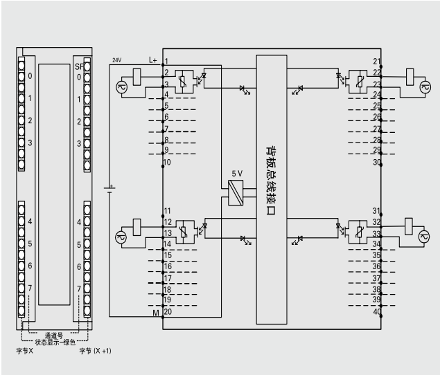
数字输出模块 SM 322 ;DO 16 x 24 /48VUC 订货号: 6ES7322-5GH00-0AB0
