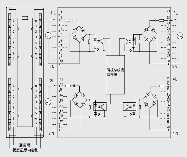
数字输入模块 SM 321 ;DI 32 × 20 VAC 订货号: 6ES7321-1EL00-0AA0
