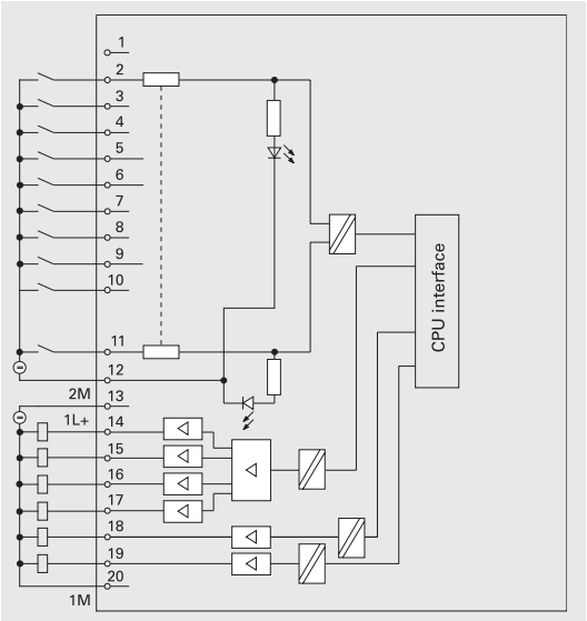
CPU 312C 内置 I/O 端子接线图
