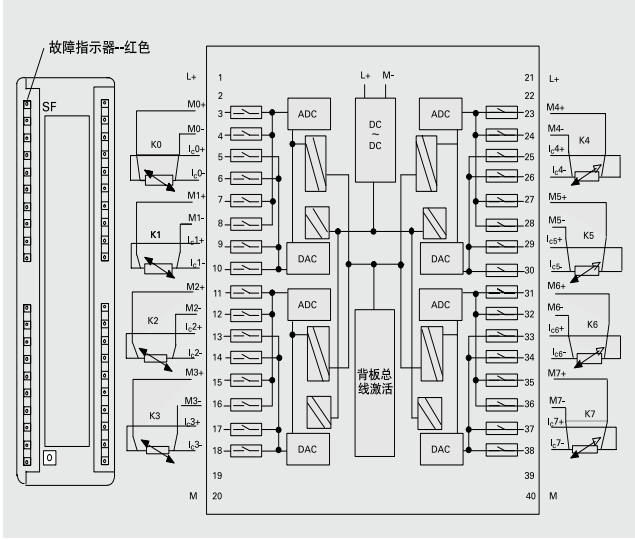
模拟量输入模块 SM 331 AI 8 x RTD 订货号: 6ES7331-7PF00-0AB0
