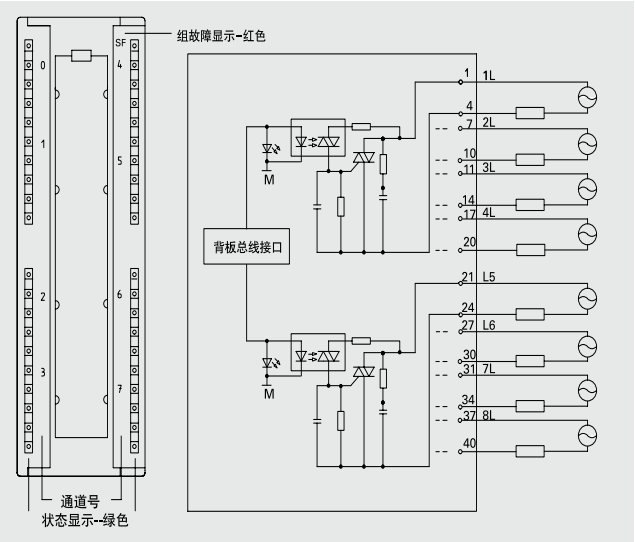
数字输出模块 SM 322; DO 8 x 120/230 VAC/2A ISOL 订货号: 6ES7322-5FF00-0AB0
