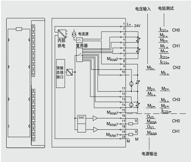
模拟量输入/输出模块 SM 334 AI 4/AO 2 x 12位 订货号: 6ES7334-0KE00-0AB0
