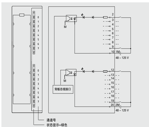
数字输入模块 SM 321 ;DI 16 x 48-125 VDC 订货号:6ES7321-1CH20-0AA0
