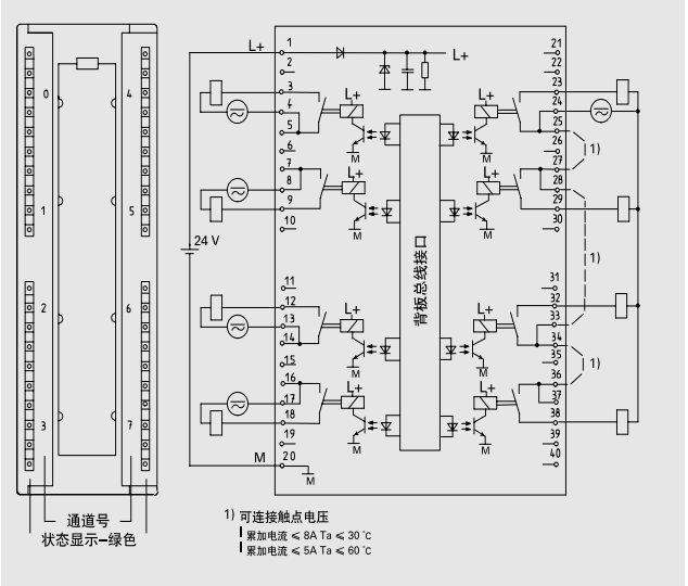
继电器输出模块 DO 8 x Rel 230 VAC/5A 订货号: 6ES7322-1HF10-0AA0
