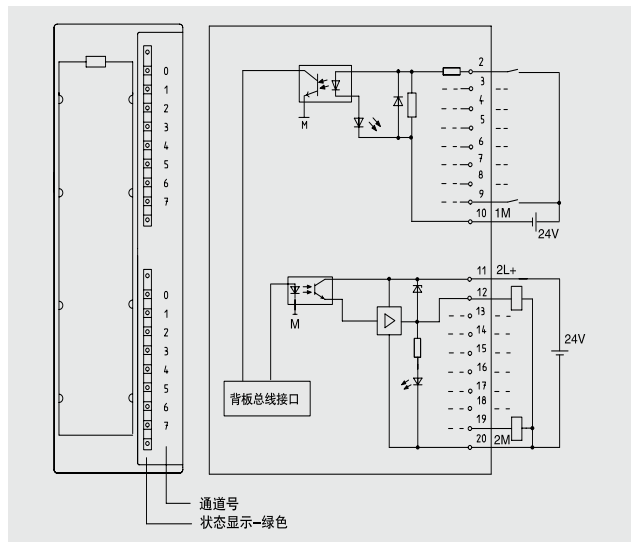
数字量输入/输出模块 SM 323 DI 8 x 24 VDC/0.5A 订货号: 6ES7322-1BH01-0AA0
