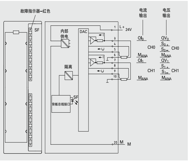
模拟量输出模块 SM 332 AO 2 × 12位 订货号: 6ES7332-5HB01-0AB0
