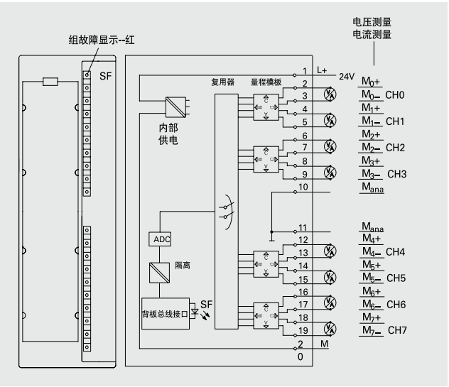
模拟量输入模块 SM 331 AI 8 x 14位 订货号: 6ES7331-7HF0x-0AB0
