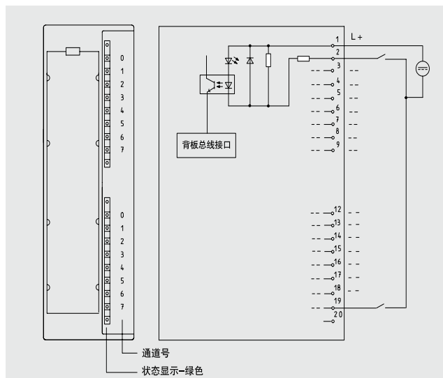
数字输入模块 SM 321 ;DI 16 x 24 VDC 订货号:6ES7321-1BH50-0AA0
