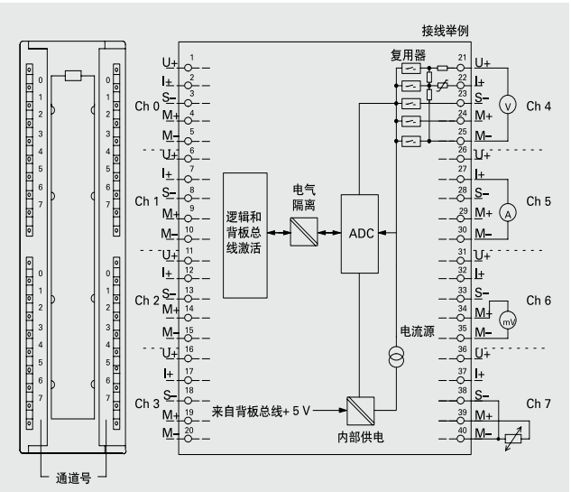
模拟量输入模块 SM 331 AI 8 x 13位 订货号: 6ES7331-7KF01-0AB0
