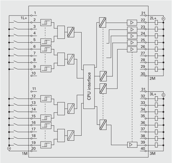
CPU 314C-2 内置 I/O 端子接线图
