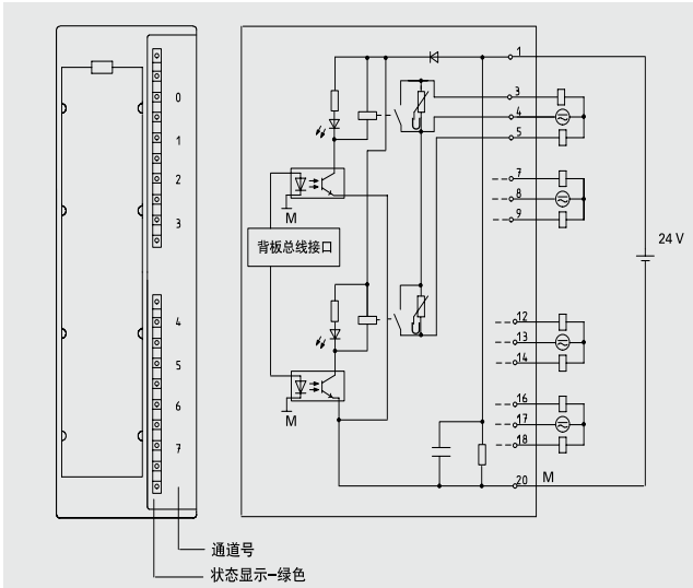
继电器输出模块 SM 322; DO 8 x REL 230 VAC 订货号: 6ES7322-1HF01-0AA0
