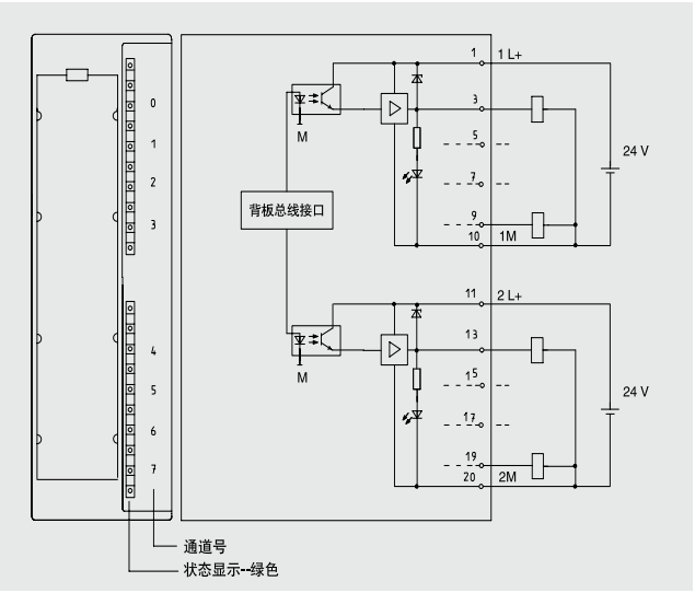
数字输出模块 SM 322; DO 8 x 24 VDC/2A 订货号: 6ES7322-1BF01-0AA0
